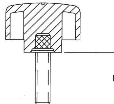
THREADED STUD
